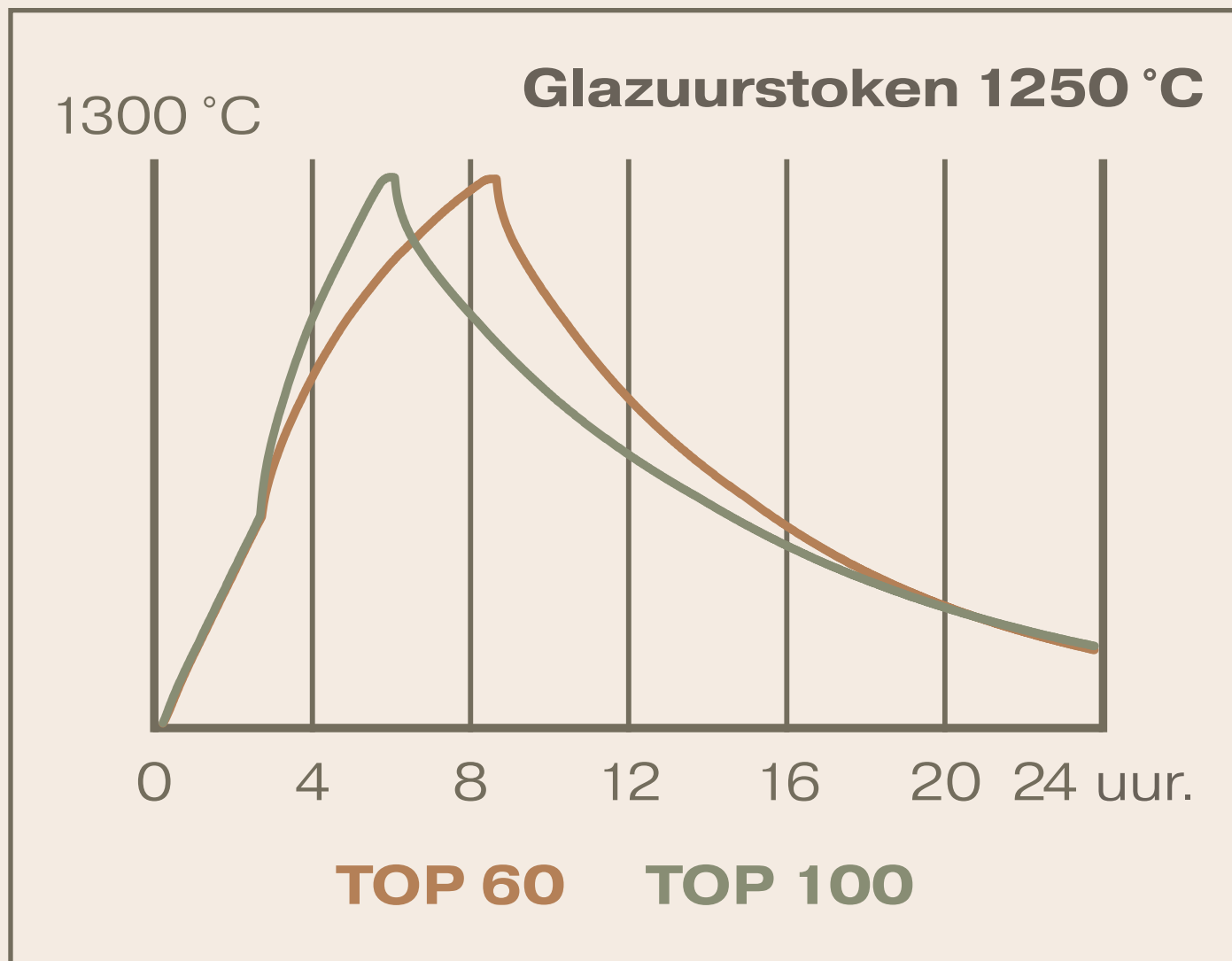
Voorbeeldcurve van een glazuurstoken
