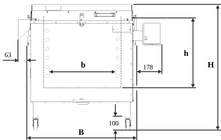
Fig5: Mått modell HO
