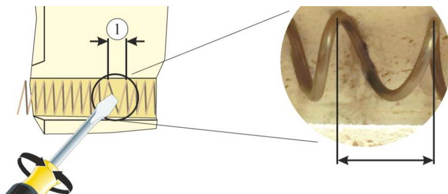
Fig. 55: Vidga värmespiralen något ((bilden är en liknande bild))
