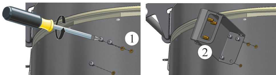
Fig. 16: Montera hållaren på ugnshuset ((bilden är en liknande bild))
