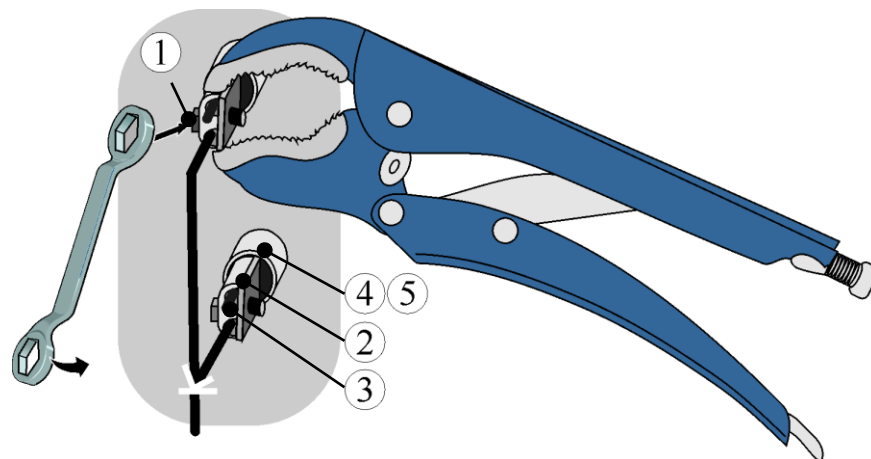
1 Sexkantskruv / 2 Anslutningsklämma / 3 Änden på värmeelementen 4 Keramik-genomföringsrör / 5 Fibervadd
