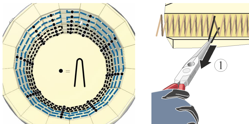
Fig. 50: Dra försiktigt ut kramporna ((bilden är en liknande bild))
