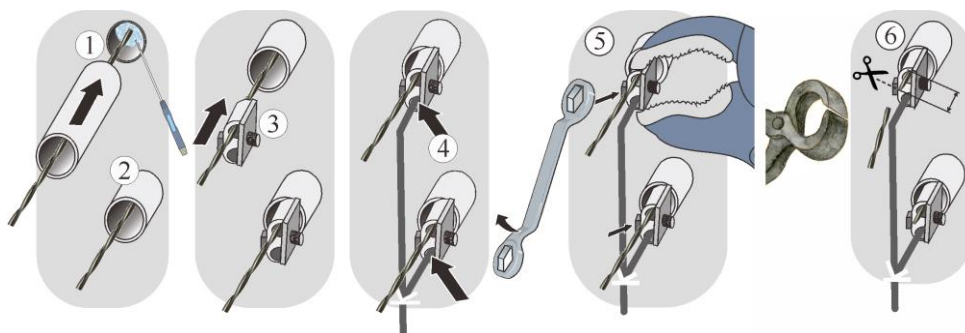
Fig. 69: Skjut på keramik-genomföringsrören och iordningställ en fackmässigt korrekt elanslutning (bilden är en liknande bild)
