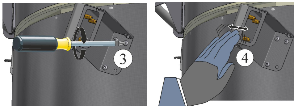
Fig. 17: Dra åt hållarens skruvar ordentligt ((bilden är en liknande bild))
