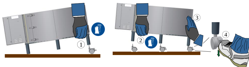
Fig14: Exempel: Montera transportrullarna på ugnar upp till 60 kg (bilden är en liknande bild)
