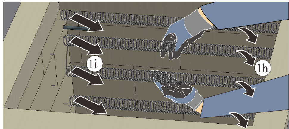
Fig. 63: Dra ut värmeelementen ur ugnsrummet (bilden är en liknande bild)
