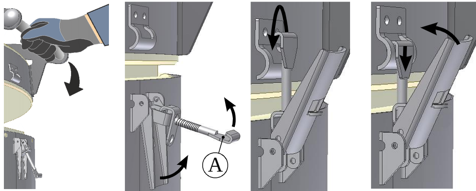
Fig. 34: Stäng lockets förslutning ((bilden är en liknande bild))
