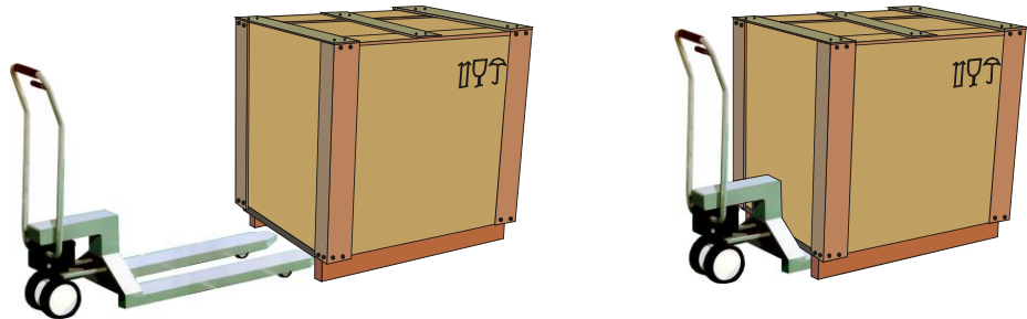
Fig7: Se till att truckens resp. lyftvagnens gafflar körs in helt och hållet under transportpallen.
