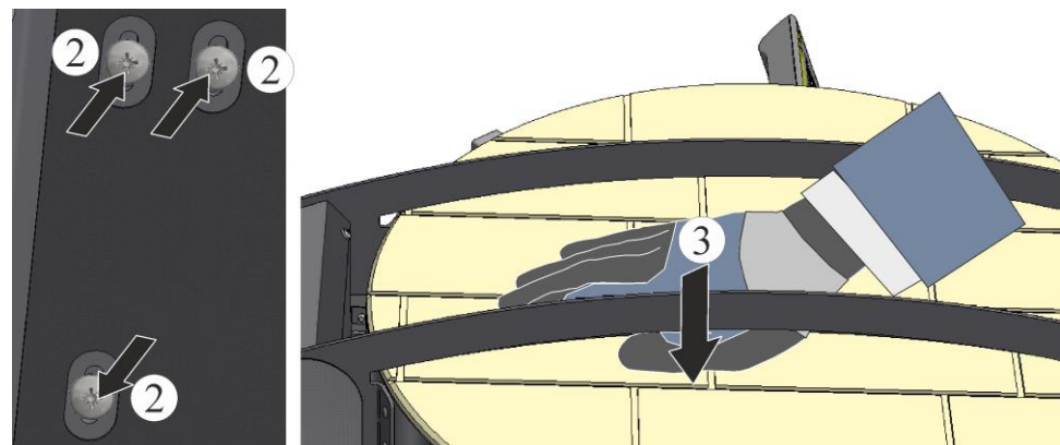
Fig. 42: Lossa skruvarna/tryck ner locket (bilden är en liknande bild)
