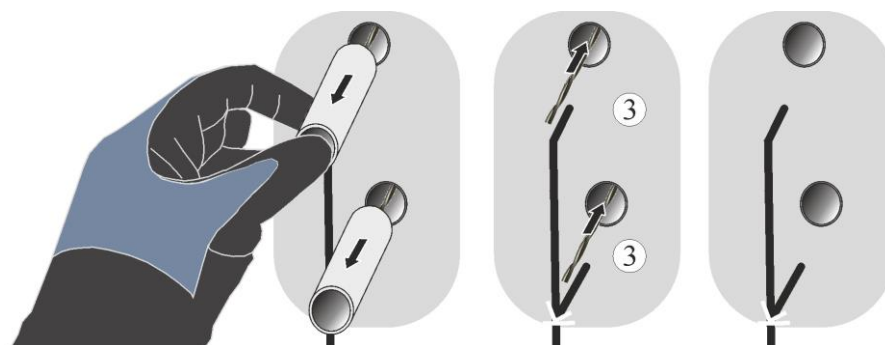
Fig. 49: Dra försiktigt ut keramik-genomföringsrören ((bilden är en liknande bild))
