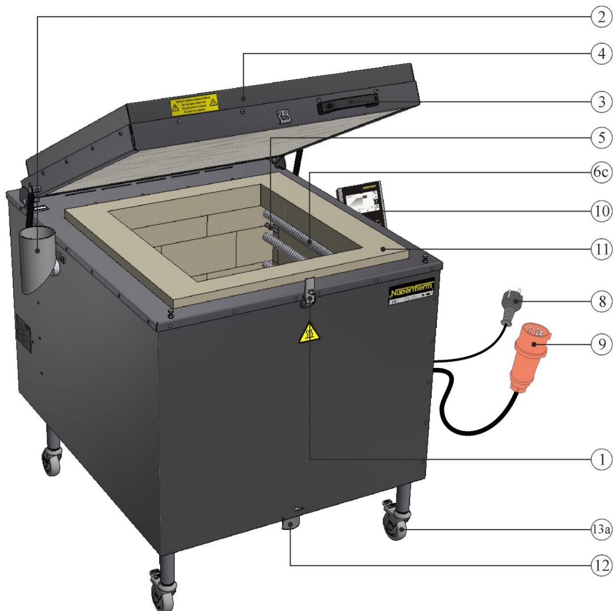
Fig2: Exempel: Toppladdare modell HO 100 (bilden är en liknande bild)
