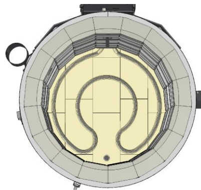
Extra utrustning zon 2 (utgång A2) (golvvärme)
