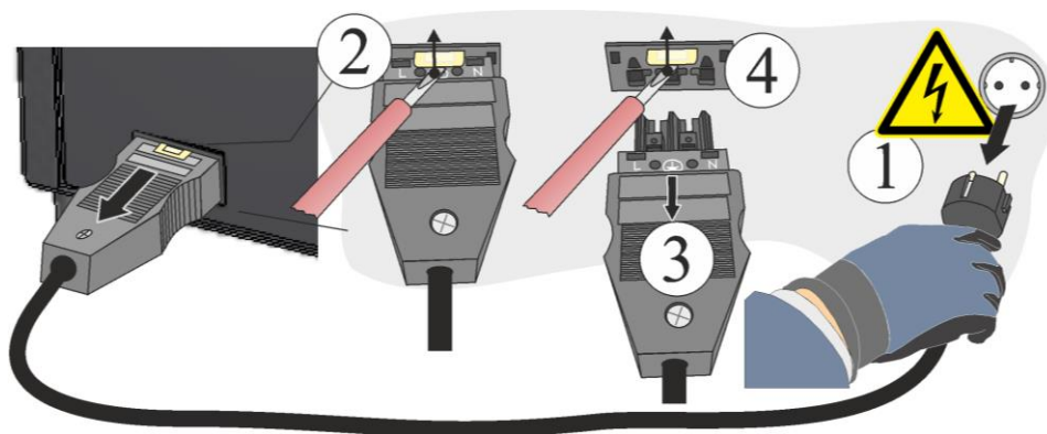
Fig44: Skilja Snap-In-kopplingen (stickkontakt) från ugnshuset (bilden är en liknande bild)
