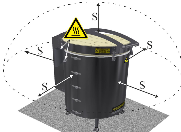
Bild 9: Minsta säkerhetsavståndet till brännbara material (liknar det på bilden)
