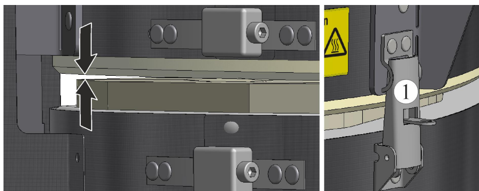
Fig40: Lås locket med låsanordningen (bilden är en liknande bild)
