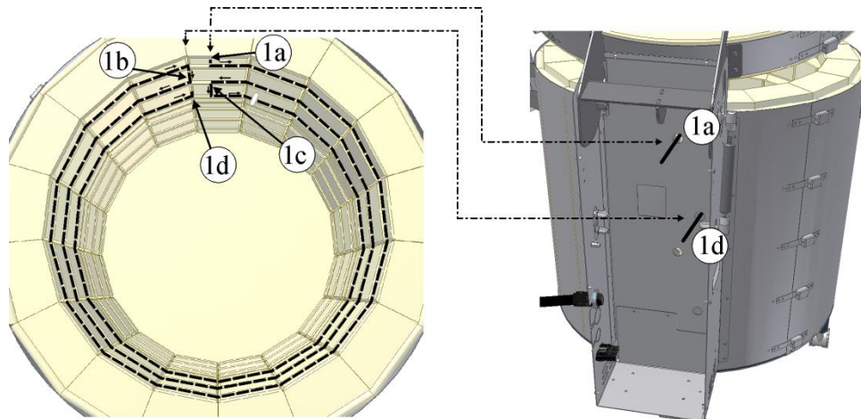
Fig. 53: Placera värmetråden i spåret runtom resp. i spåren runtom ((bilden är en liknande bild).
