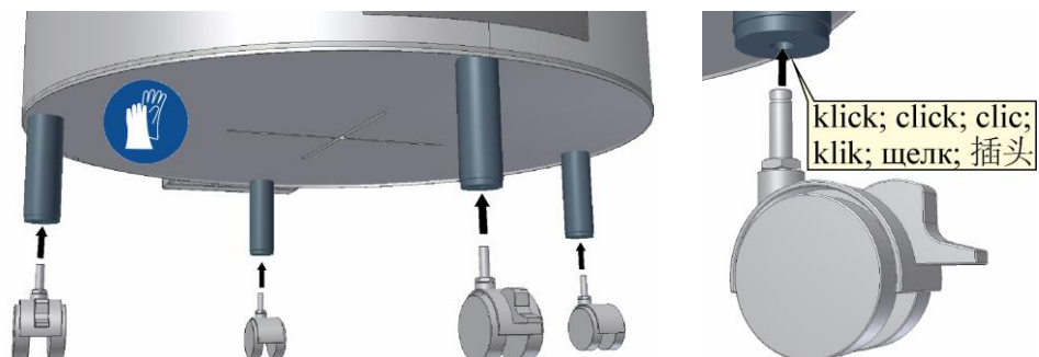
Fig12: Montera transportrullarna (bilden är en liknande bild)
