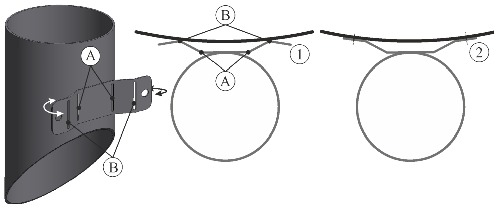
Fig. 20: Anpassa bypass-stosens hållare ((bilden är en liknande bild))
