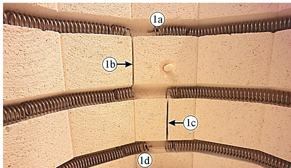
Fig. 54: Placera värmetråden i spåret runtom resp. i spåren runtom ((bilden är en liknande bild)
