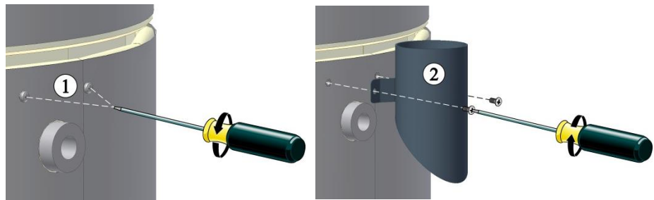
Fig21: Montera bypass-stosen (bilden är en liknande bild)
