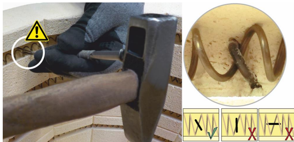
Fig. 57: Så slår du in kramporna i isoleringen ((bilden är en liknande bild)
