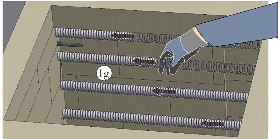
Fig. 62: Dra u bärrören (1g) (bilden är en liknande bild)
