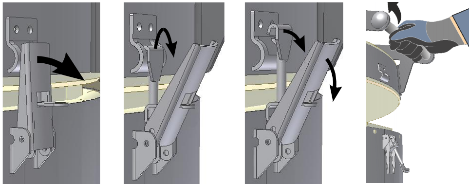
Fig33: Öppna lockets låsanordning (bilden är en liknande bild)
