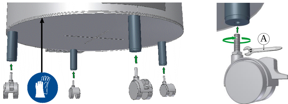
Fig13: Montera transportrullarna (bilden är en liknande bild)
