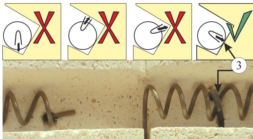
Fig. 56: Krampornas rätta positionering ((bilden är en liknande bild))
