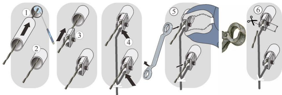
Fig. 58: Skjut på keramik-genomföringsrören och iordningställ en fackmässigt korrekt elanslutning (bilden är en liknande bild)
