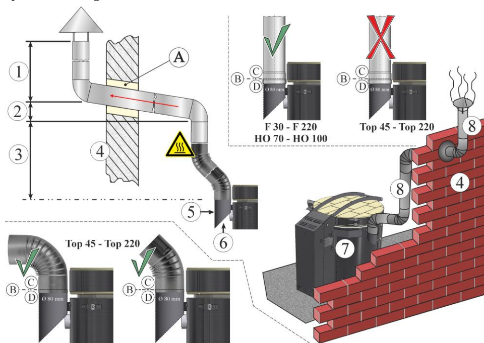
Fig23: Exempel: Montera frånlufrören (bilden är en liknande bild)
