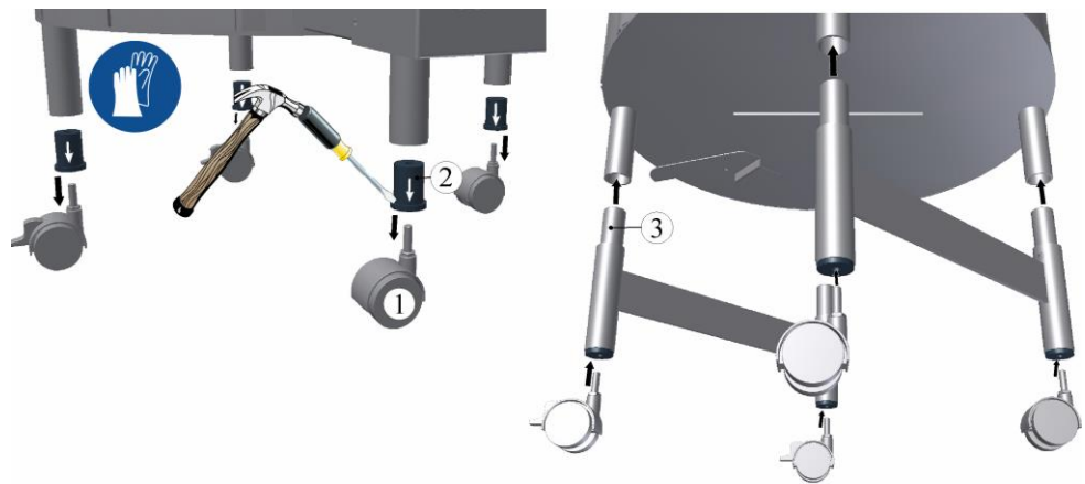
Fig11: Montera den högre stommen (bilden är en liknande bild)
