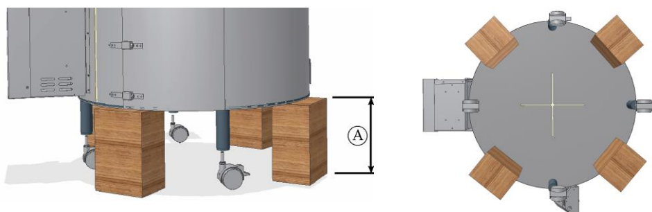
Fig15: Exempel: Montera transportrullarna på ugnar som väger mer än 60 kg (bilden är en liknande bild)
