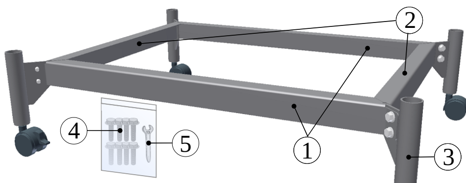
Fig10: Stommens enskilda delar (bilden är en liknande bild)
